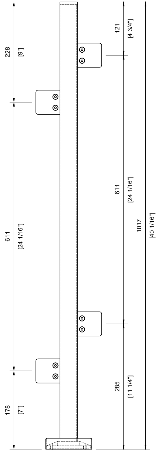
#SSPEFT36SL Scale: 1:5
