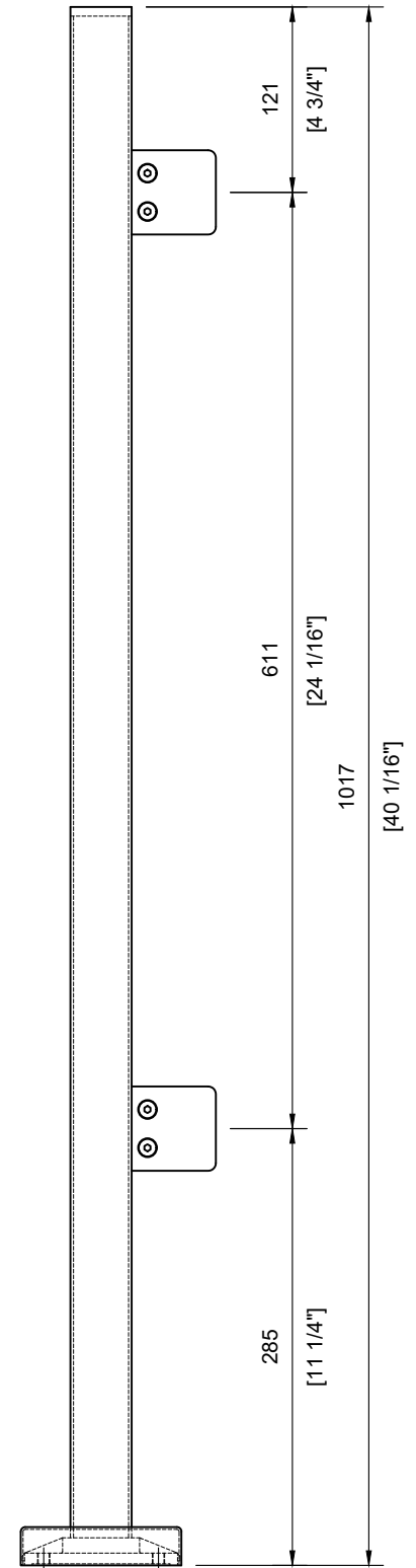
#SPEFT36SBE Scale: 1:5
