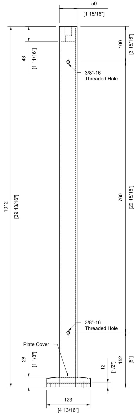
#SSHPSQR50E Scale: 1:5
