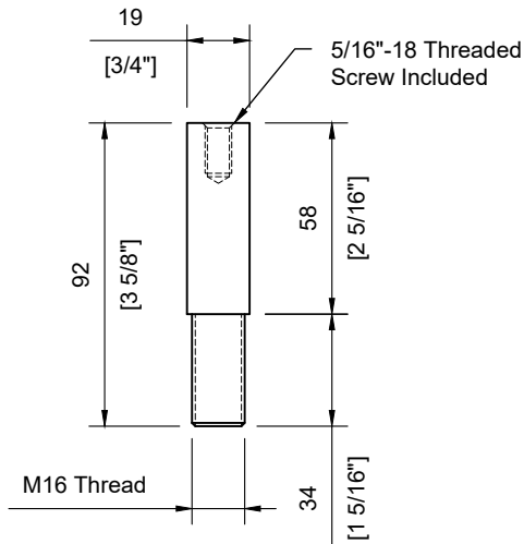
#SSHPZAC01 Scale: 1:2
