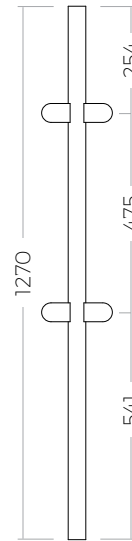
SSPG166X42L Line Post 42"
