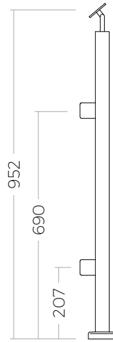
⑧ SSPE36STEM End
