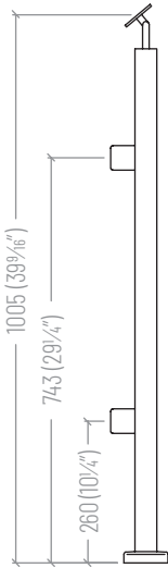
STAIR END - Back ⑨ SSPE36STEB
