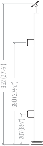
STAIR END - Middle ⑧ SSPE36STEM
