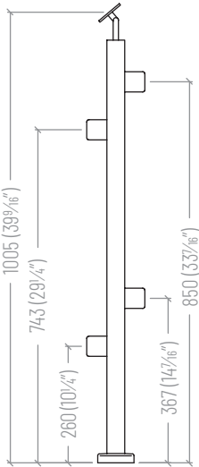
STAIR LINE - Back ⑥ SSPE36STLB
