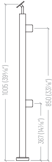
STAIR BOTTOM - Back ③ SSPE36BPB
