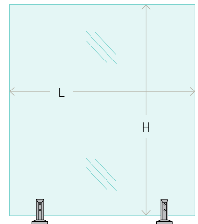
Profil de verre affichant le travail de la bordure
