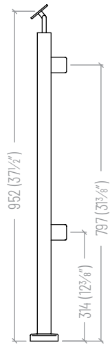
ESCALIER - POTEAU DU BAS - Milieu
