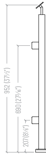
ESCALIER - POTEAU DE FIN - Milieu
