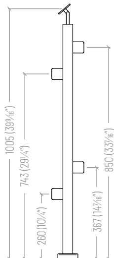
ESCALIER - POTEAU EN LIGNÉ - Arrière
