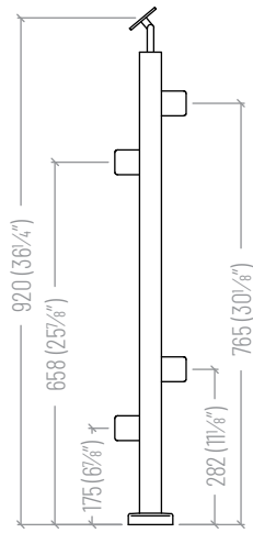
ESCALIER - POTEAU EN LIGNÉ - Avant
