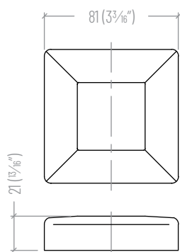
COUVERT D'EMBASE
