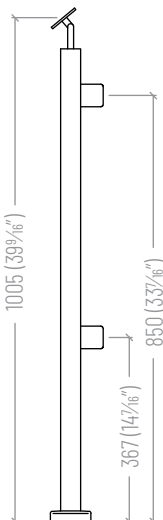
ESCALIER - POTEAU DU BAS - Arrière
