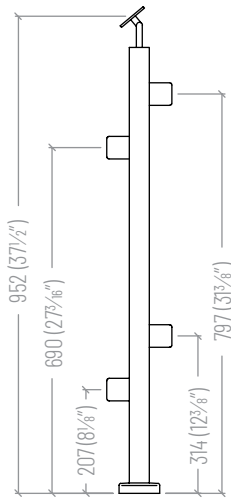
ESCALIER - POTEAU EN LIGNÉ - Milieu
