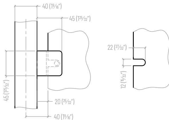
PINCE POUR VERRE
