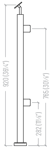
ESCALIER - POTEAU DU BAS - Avant
