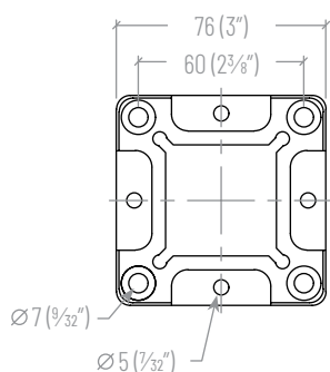
PLAQUE D'EMBASE
