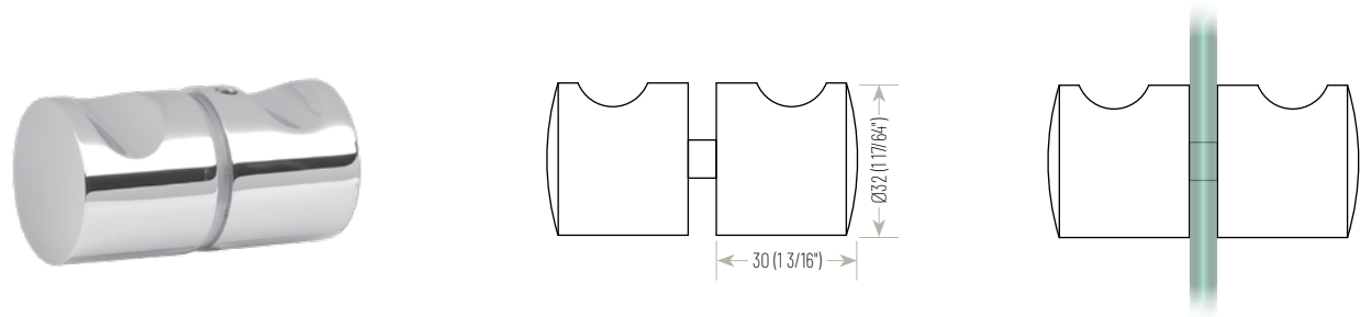
SSSFDK1 • ROUND Modern Knob
