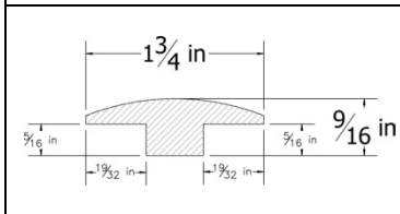
9/16" x 1 3/4" T-MOULD
