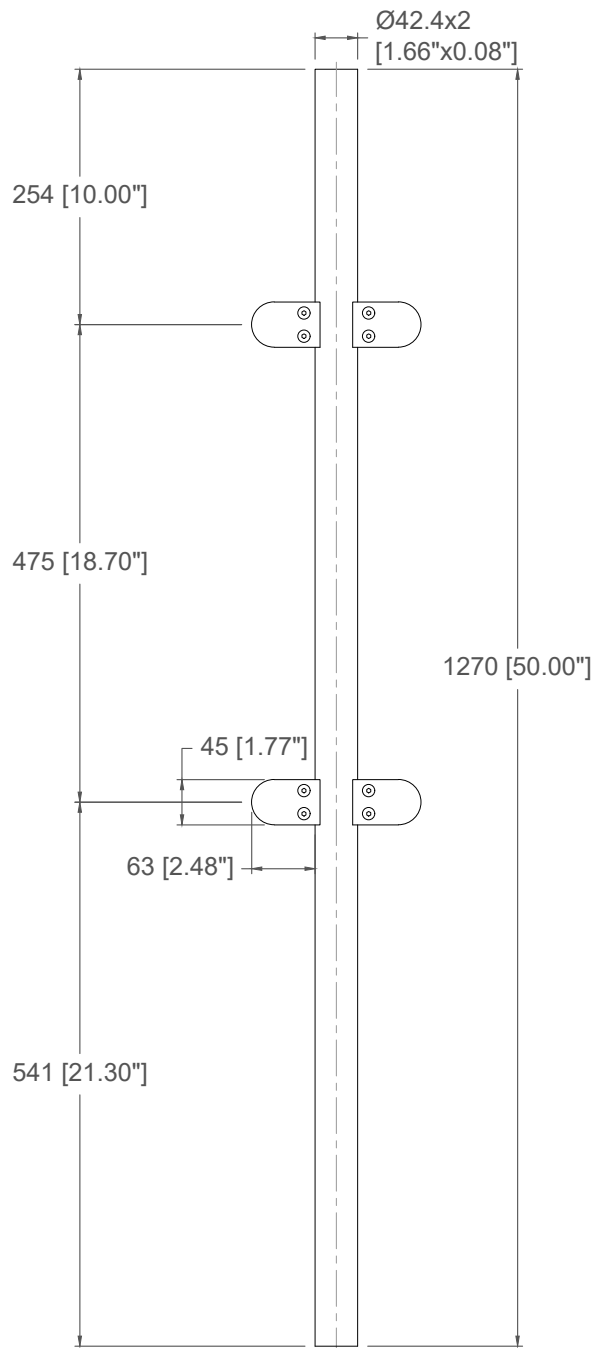
Line Post: SSPG166X42L
