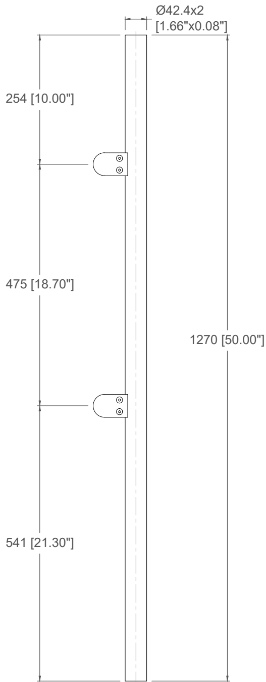
End Post: SSPG166X42E
