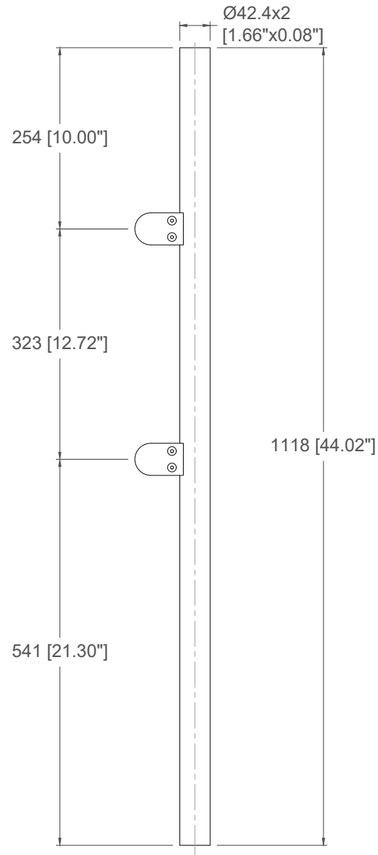
End Post SSPG166X36E
